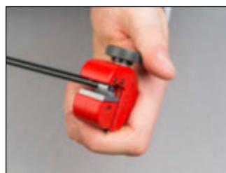
Poloha vedení pro oškrabání opláštění
