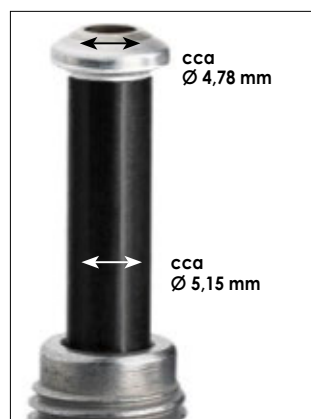
Poloha vedení pro oškrabání opláštění
