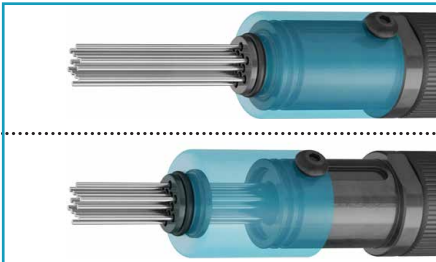
Nastavitelné jehlové saně s integrovaným vedením jehly zaručují dlouhou životnost
