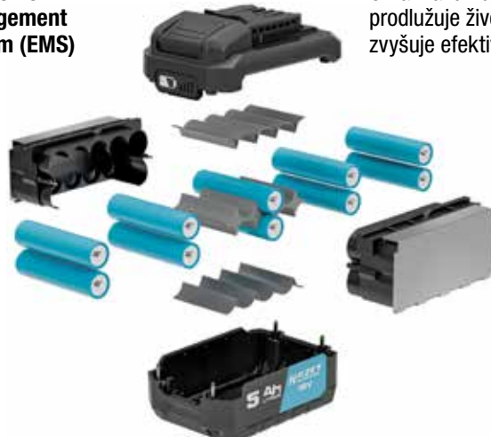
Akumulátor s patentovanou technikou Thermatec®: Integrovaný chladič systém k prodloužení životnosti
